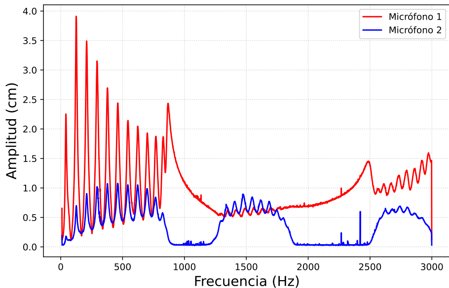
Figura 2: Datos de los micrófonos.
