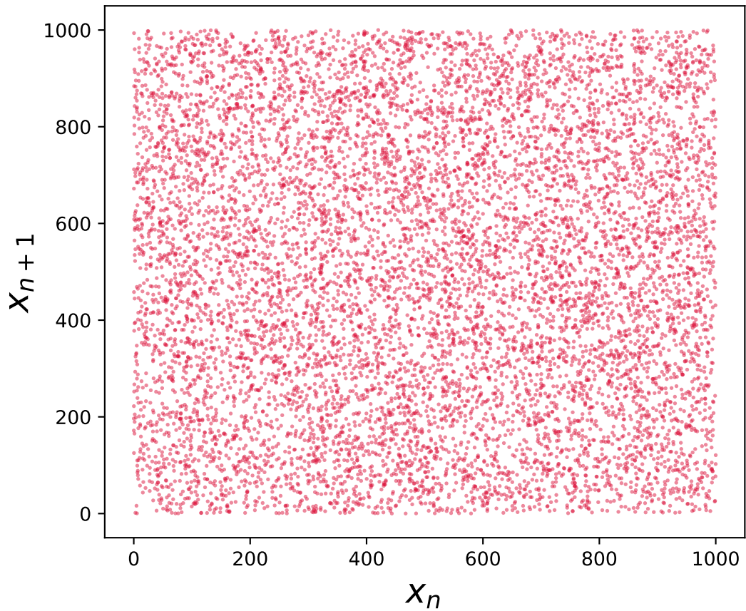
Correlación x_n vs x_{n+1} (A mano - LCG)
