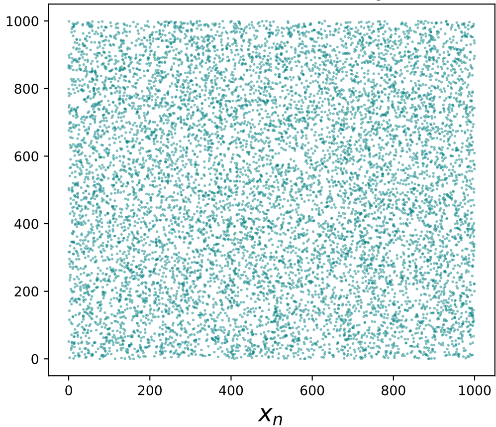
Correlación x_n vs x_{n+1} (NumPy - PCG64)
