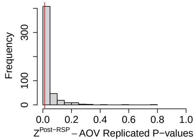
(d) HNB Linear, Z^{\text{Post-RSP}} - AOV P-values
