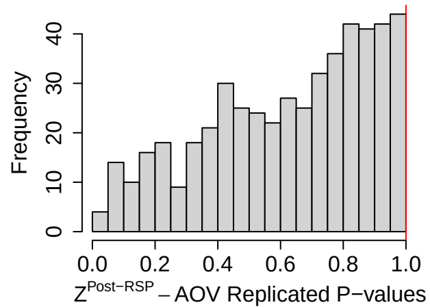
(d) HNB Nonlinear, Z^{\text{Post-RSP}} - AOV P-values
