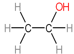
エタノールの化学構造
