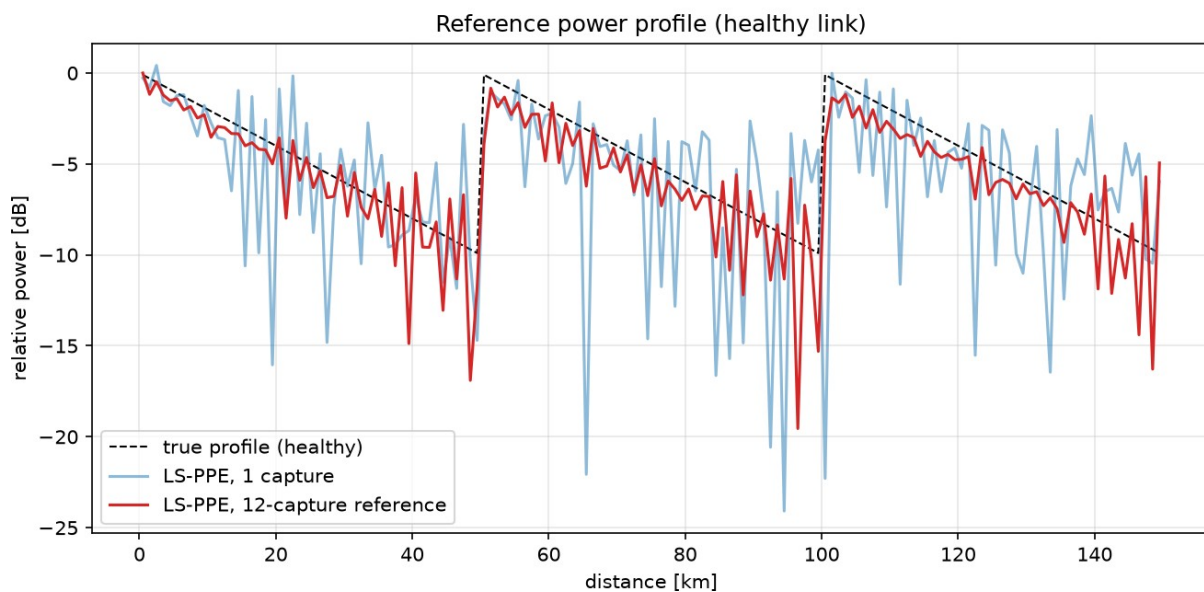
图 1 健康链路功率轮廓：单次采集 LS-PPE（蓝）噪声显著；12 次平均（红）作为参考轮廓，三跨锯齿结构清晰。
