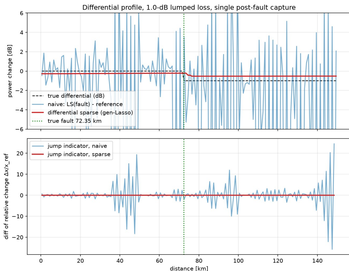
图 2 1 dB 集总损耗、单次故障后采集。上：朴素相减（蓝）被噪声淹没，差分稀疏解（红）为干净阶跃，位置正确（幅度受 Lasso 收缩，见 5.3 重拟合）；下：稀疏跳变指示仅在故障格点非零，朴素指示噪声跳变遍布全链。
