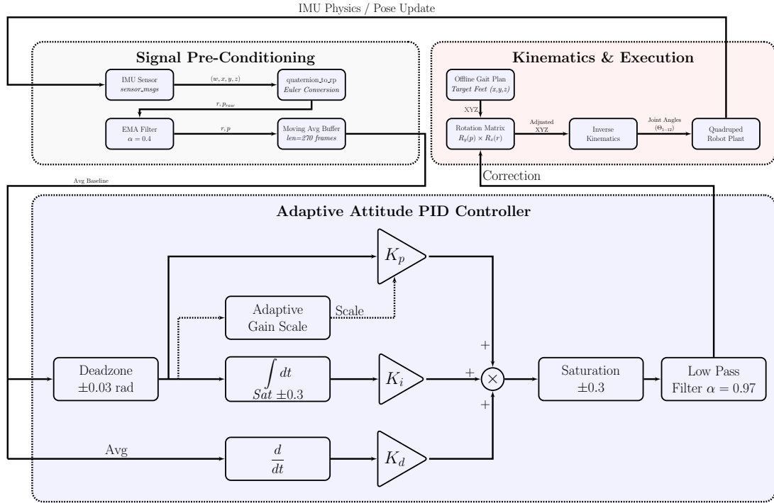
Hình 2-25: Kiến trúc bộ điều khiển PID thích nghi cho ổn định tư thế
