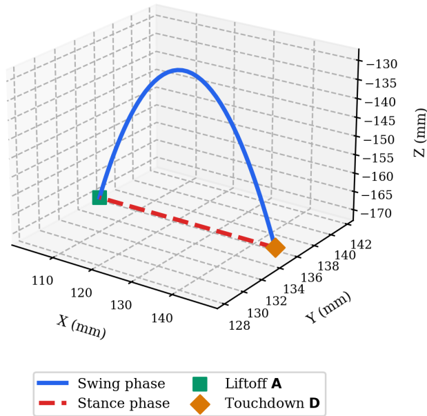
Hình 5-6: Quỹ đạo 3D bàn chân chân trước bên trái trên hệ thống mô phỏng
