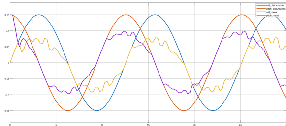
Hình 29: Đáp ứng hàm Sine với K_p=1 , K_i=0 , K_d=0
