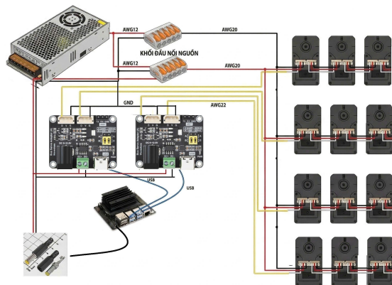
Hình 11: Sơ đồ hệ thống dây điện tổng thể
