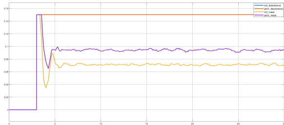
Hình 28: Đáp ứng hàm Step với K_p=1 , K_i=0 , K_d=0
