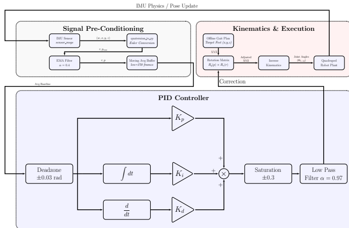
Hình 14: Sơ đồ chuỗi xử lý tín hiệu PID 5 giai đoạn
