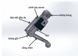
Hình 7: Cụm khớp hông (trái) và cấu trúc một chân (phải)
