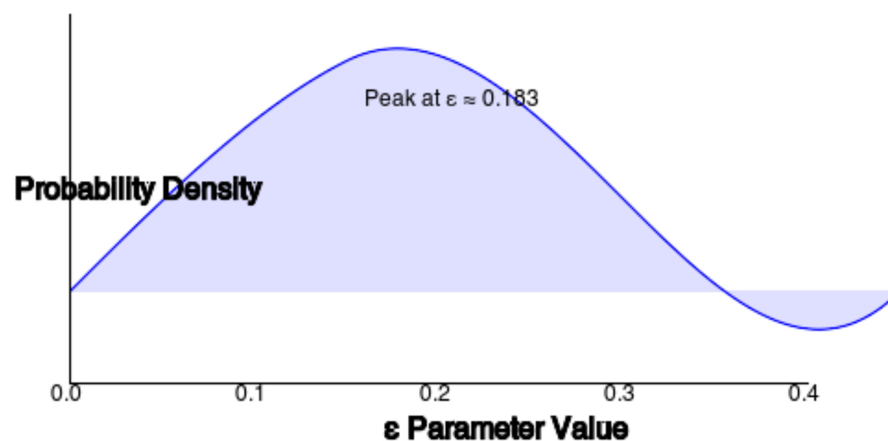
(a) Posterior Distribution of \varepsilon
