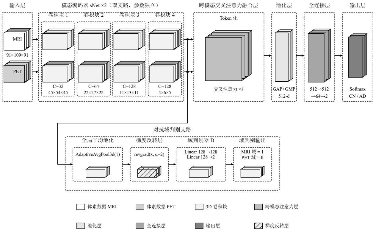
图 1 TransMF 多模态融合网络结构与数据流
