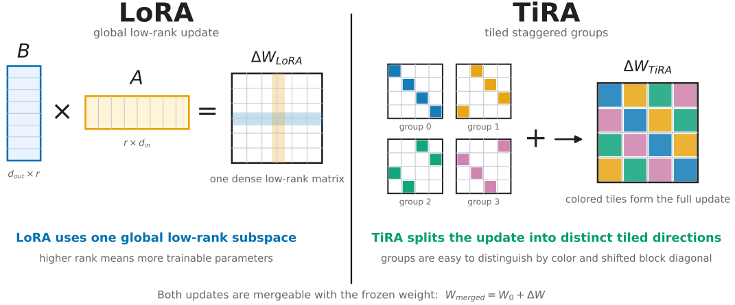
图 1: LoRA 与 TiRA 架构对比。LoRA 通过低秩分解 BA 构造权重增量 \Delta W ，其秩上限为 r ；TiRA 将 \Delta W \in \mathbb{R}^{d \times d} 划分为 M \times M 的块网格，利用 K 组可训练短向量通过外积生成秩-1 子块，并沿 K 条错位块对角线结构化填充。其中 W_0 为冻结的原始权重， K 与 M 为 TiRA 的核心超参数，控制参数分组与分块粒度。
