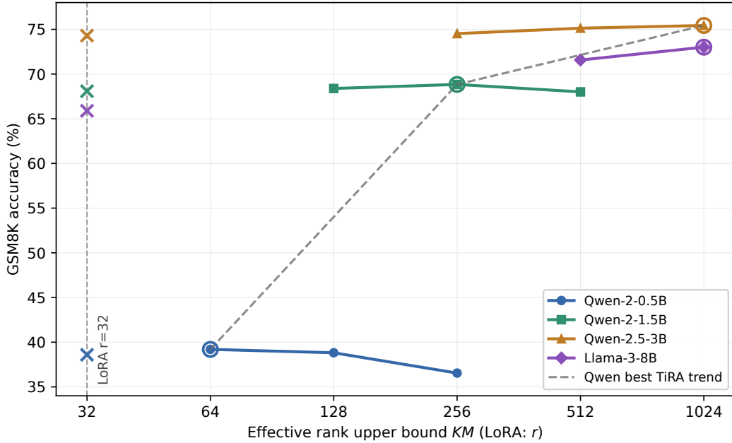
图 3: 固定 K = 32 时，不同模型在 LoRA 与 TiRA 不同分块粒度下的 GSM8K 准确率变化。横轴为有效秩上限；LoRA ( r = 32 ) 以叉号标在横轴 32 处。空心圆标出各模型上 TiRA 的最优配置，灰色虚线连接 Qwen 系列模型的最优 TiRA 点以突出最优分块粒度随模型规模增大的右移趋势。
