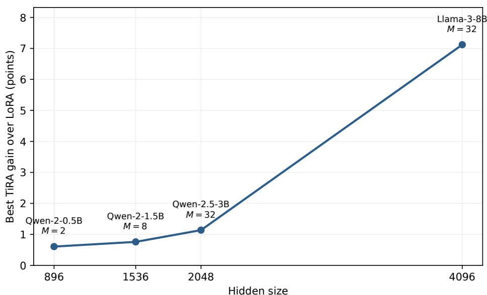
图 4: 不同模型规模下最佳 TiRA 配置相对 LoRA ( r = 32 ) 的准确率增益。横轴为隐藏维度，纵轴为最佳 TiRA 与 LoRA 的 GSM8K 准确率差值。点旁标注对应模型在当前搜索范围内的最优分块粒度 M 。
