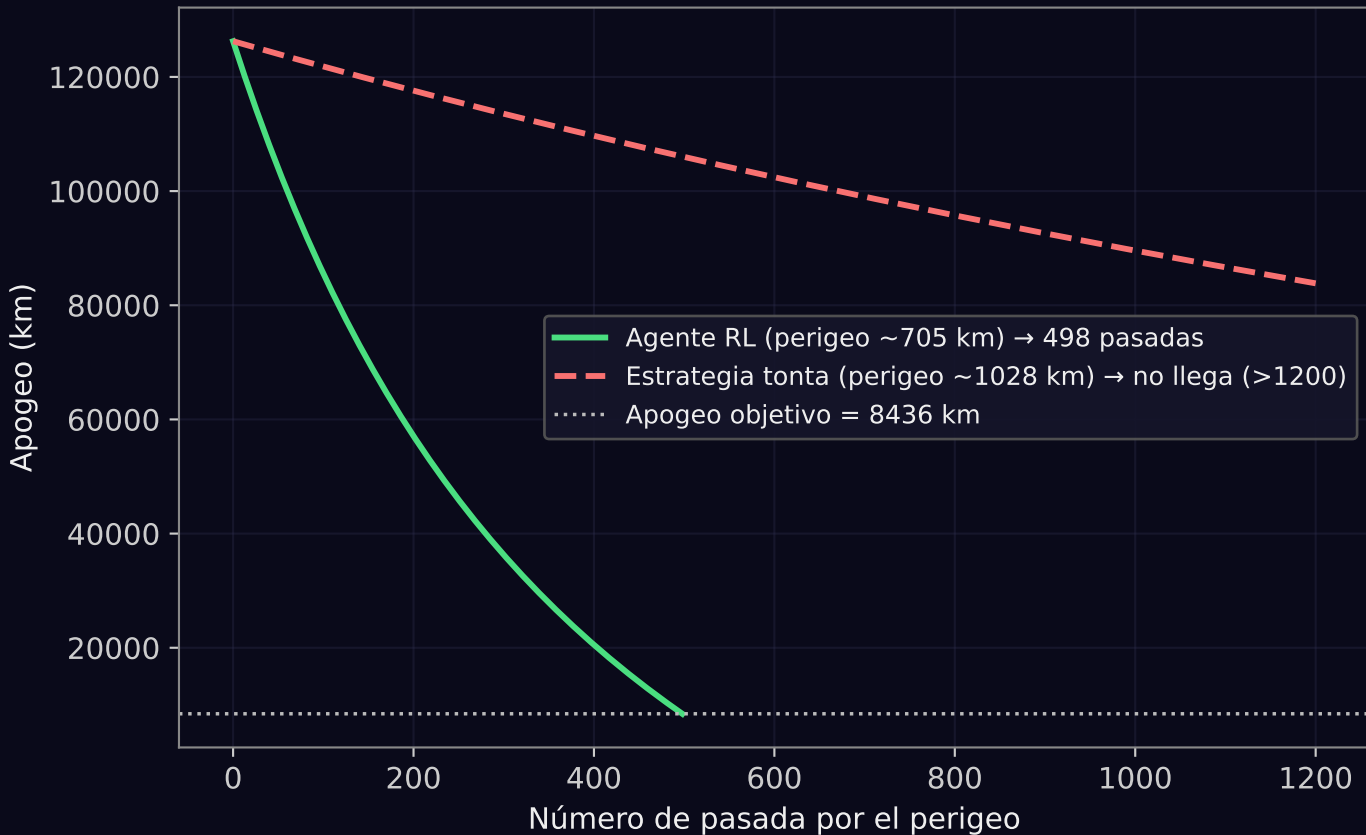
Jupiter: agente RL vs estrategia tonta (perigeo alto fijo)
