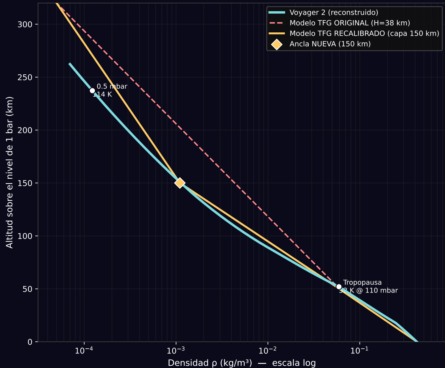
A) Perfil de densidad: modelo vs Voyager 2
