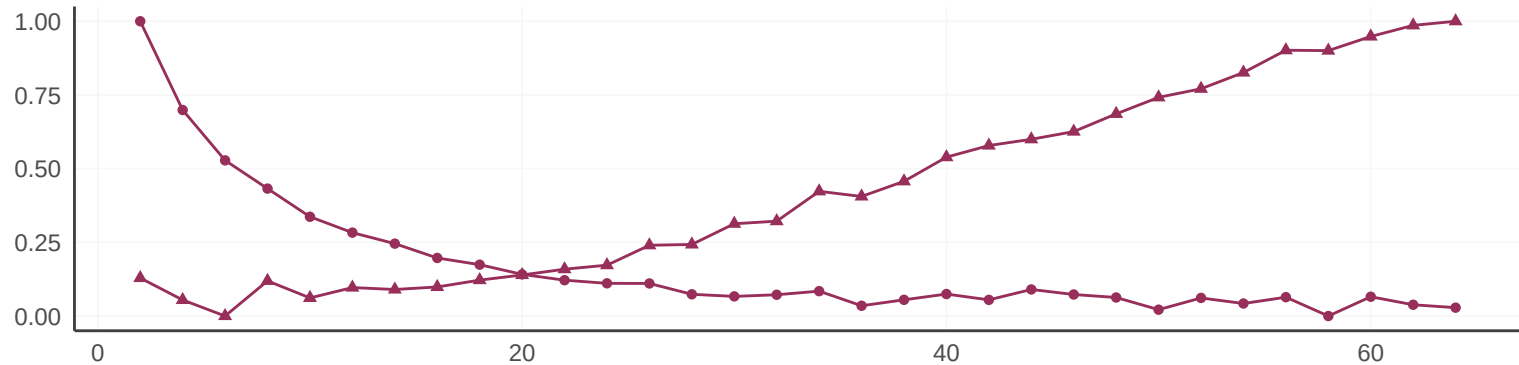
Maximise
