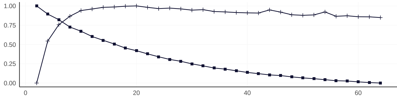
Maximise
