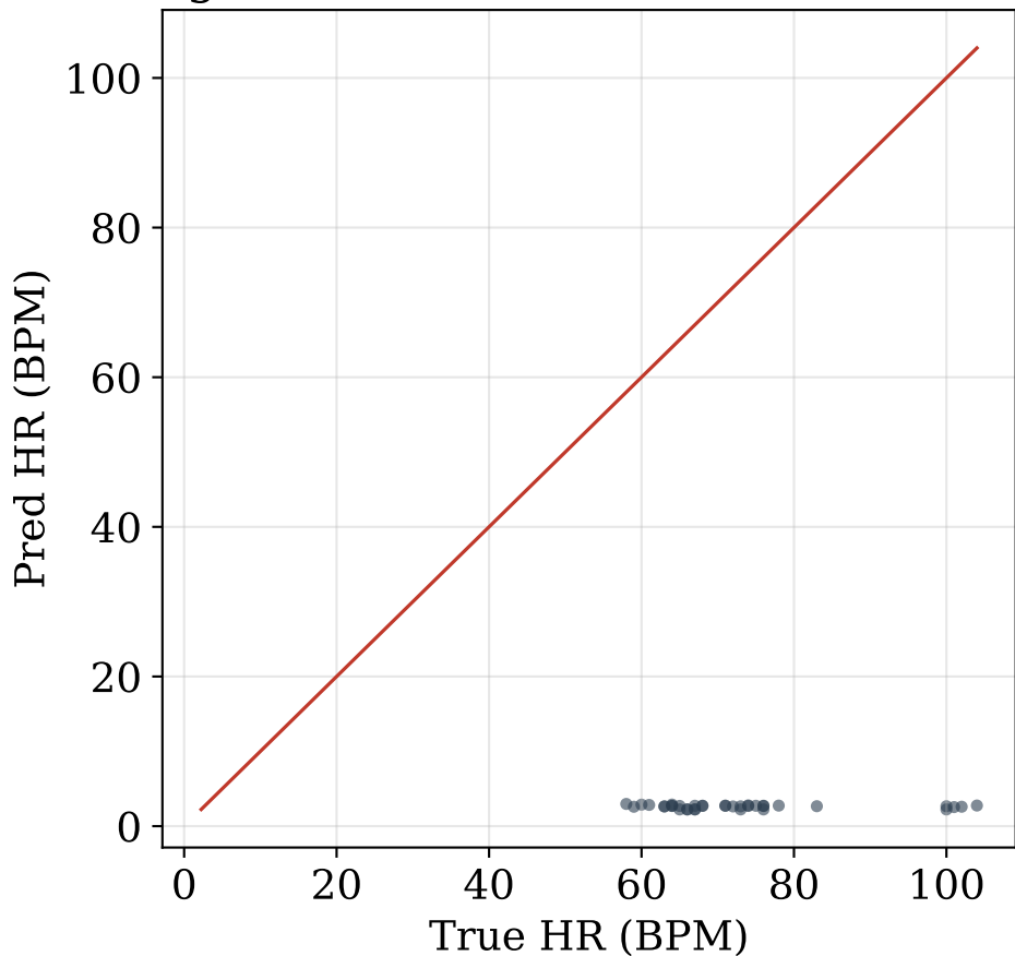
Fig.X Cross-domain HR Probe (BUT)
