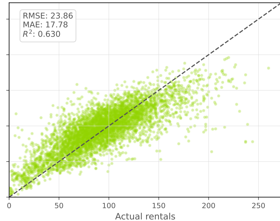
Lasso
