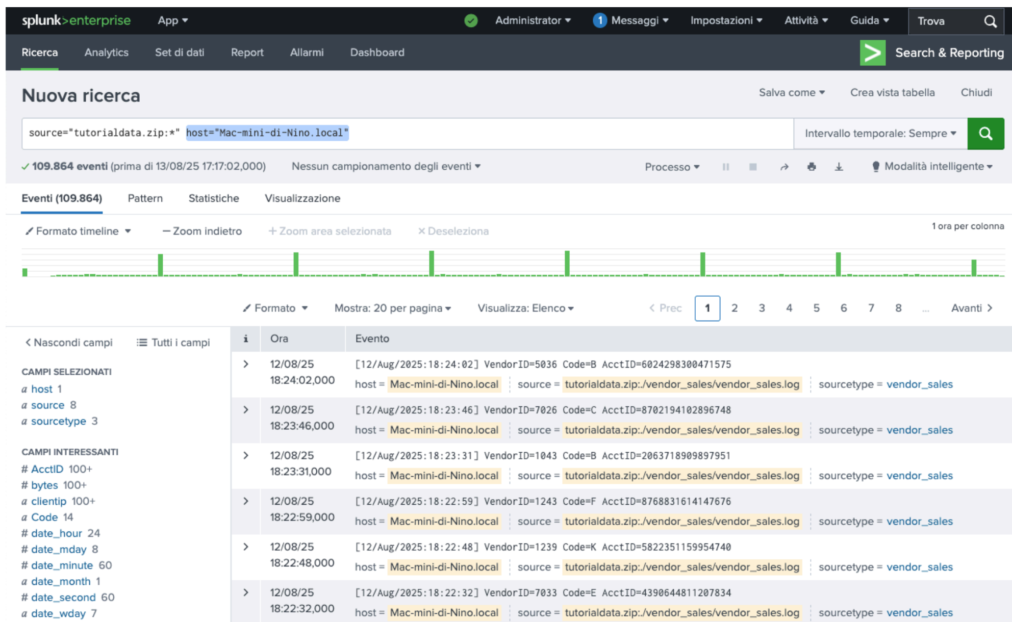
Interfaccia Splunk
