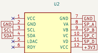
MCP4728 (Adafruit 4470)
