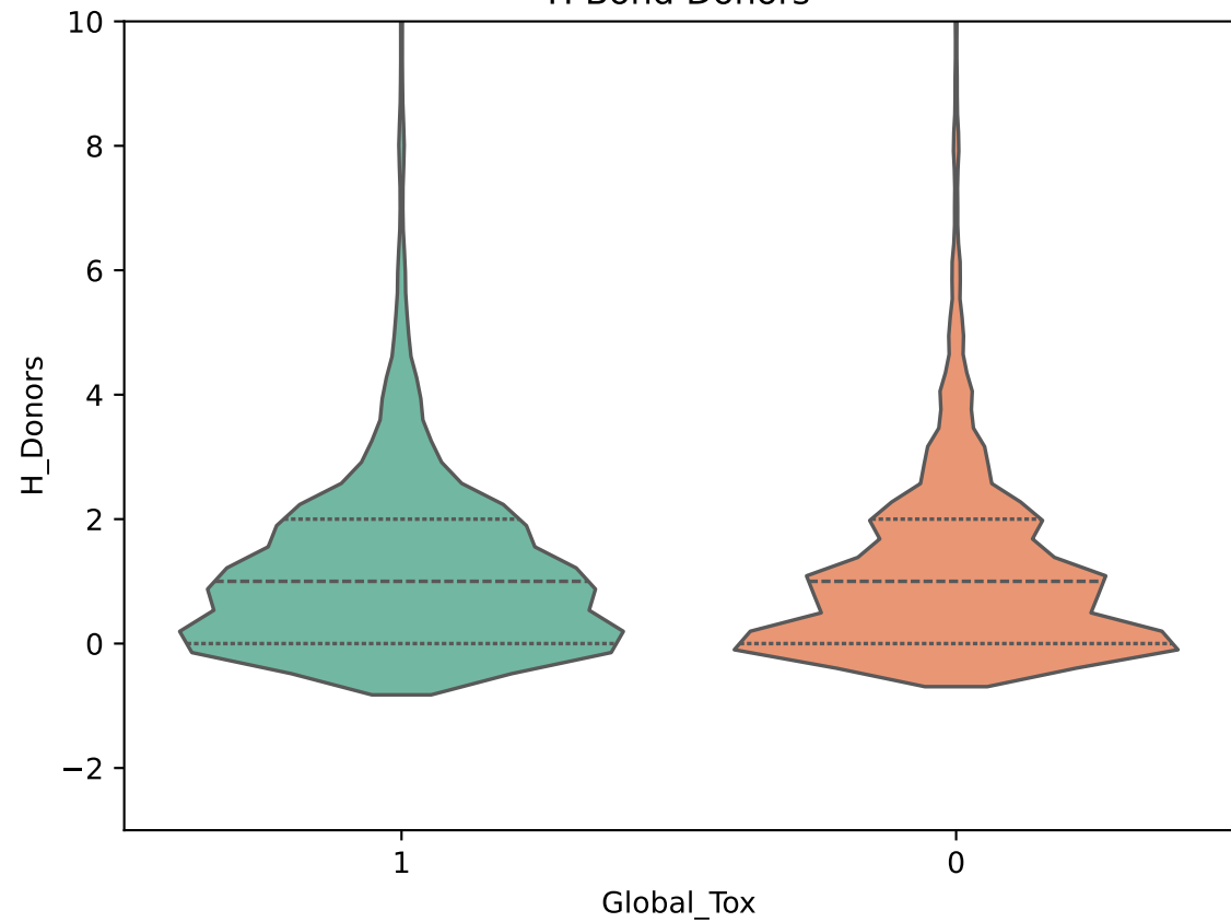
H-Bond Donors
