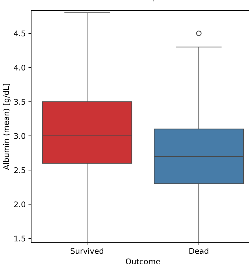
Albumin (mean) vs Outcome
