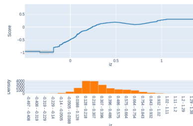
Term: iz (continuous)
