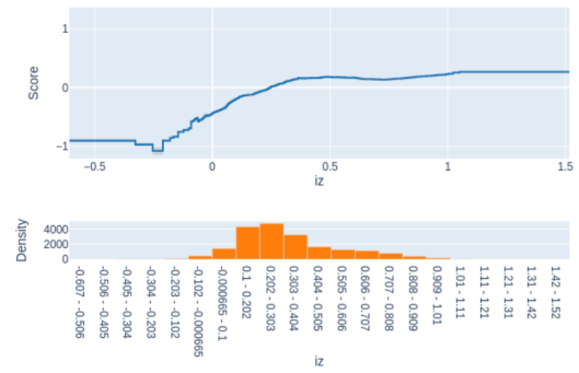
Term: iz (continuous)
