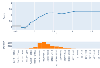
Term: iz (continuous)
