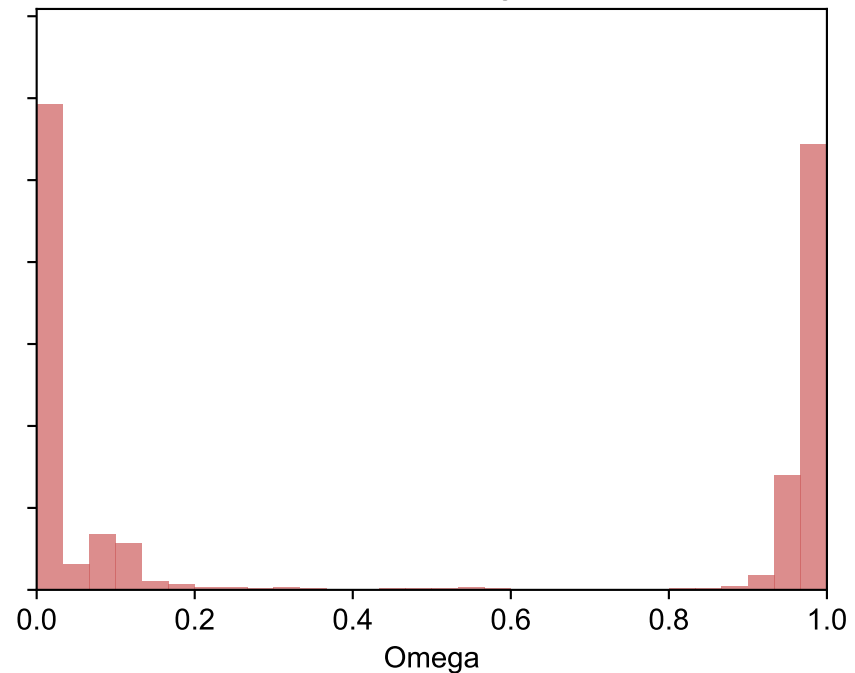
BUIP - Emergent
