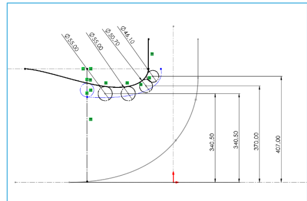
Figura 8 Tubo di flusso 4
