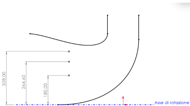
Figura 3 Linee di corrente
