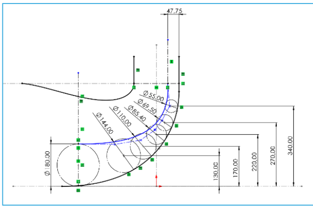
Figura 5 Tubo di flusso 1
