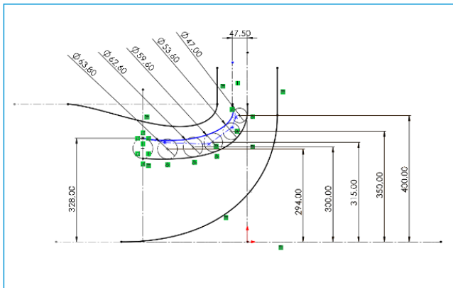
Figura 7 Tubo di flusso 3
