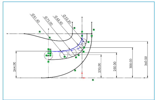
Figura 6 Tubo di flusso 2
