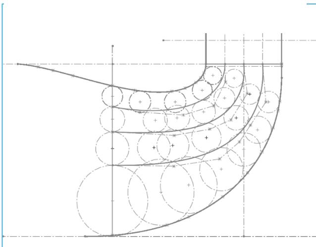
Figura 9 Tubi di flusso
