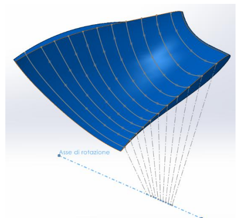
Figura 31 Distribuzione dei Theta da CAD
