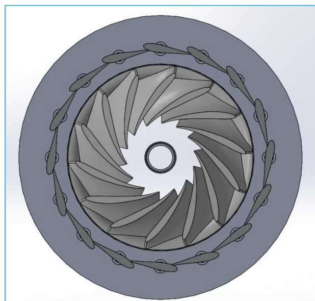
Figura 21 Distributore con pale in completa chiusura
