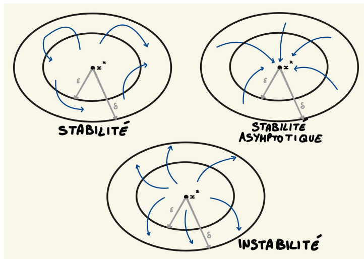
FIGURE 5.1 – Stabilité, Stabilité asymptotique, Instabilité
