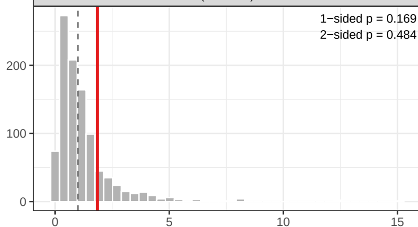
MaleUnique_Down (Males)
