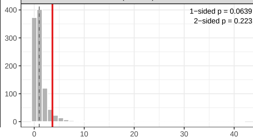
MaleUnique_Up (Males)
