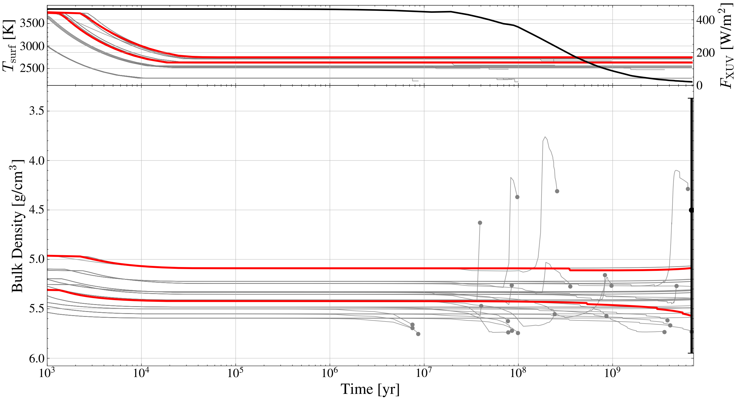
TOI1416
