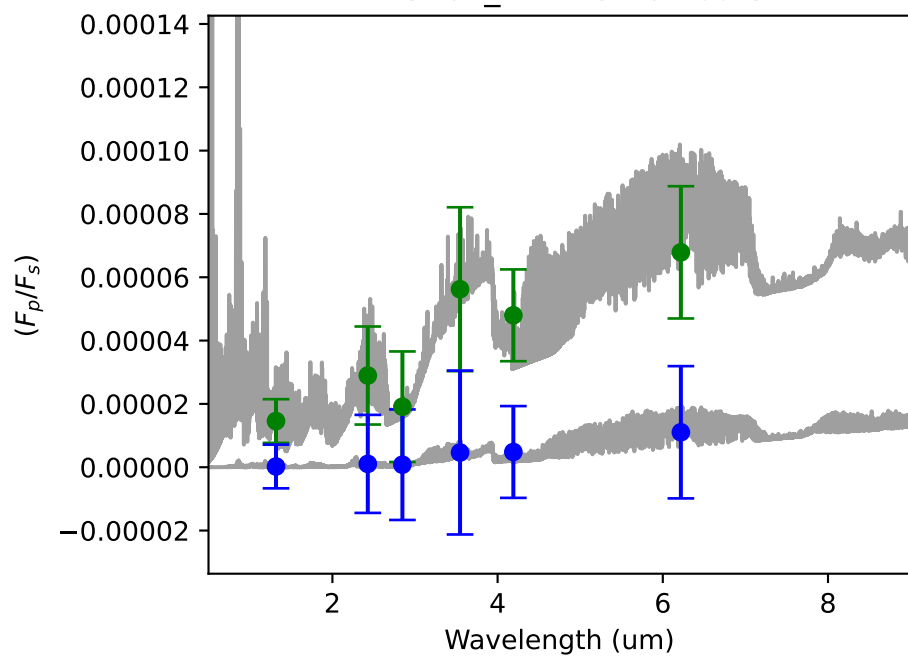
LHS1478_1 - 234.00 hours
