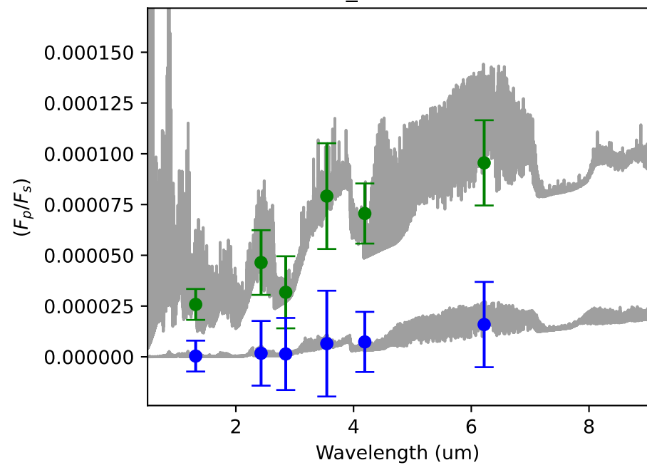
TOI561_1 - 54.00 hours
