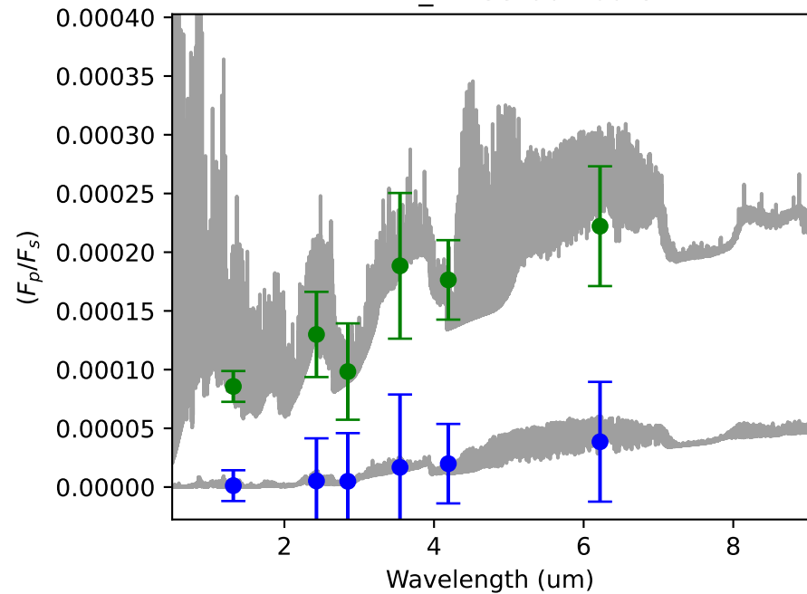
TOI431_1 - 58.80 hours
