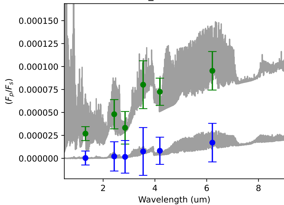
TOI561_10 - 54.00 hours
