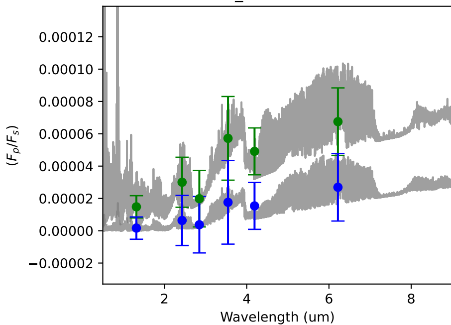
LHS1478_10 - 234.00 hours
