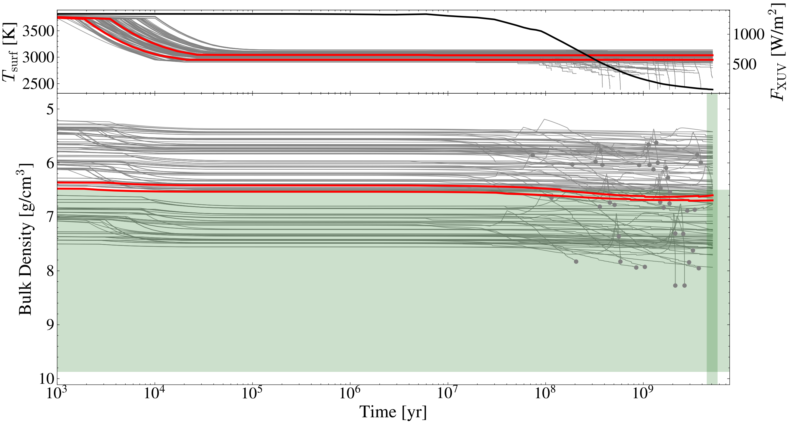
TOI431
