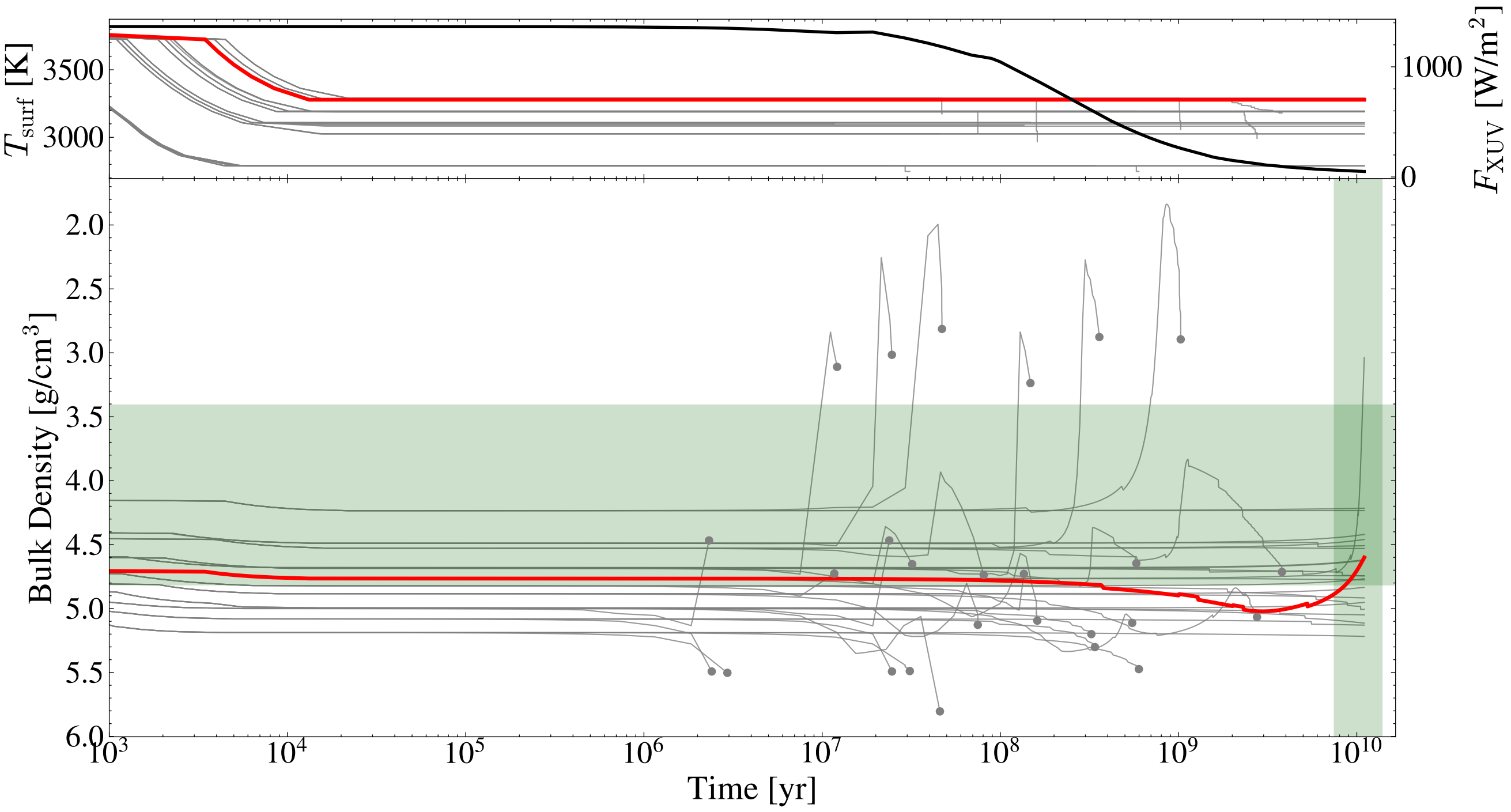
TOI561
