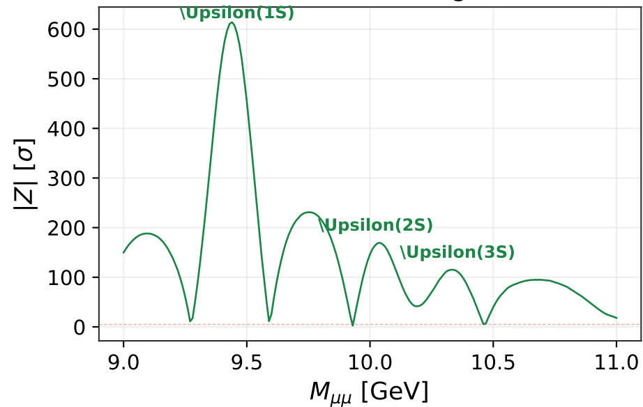
Bottomonium Region
