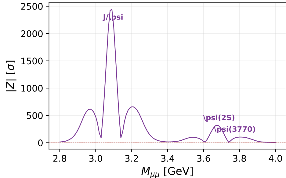
Charmonium Region
