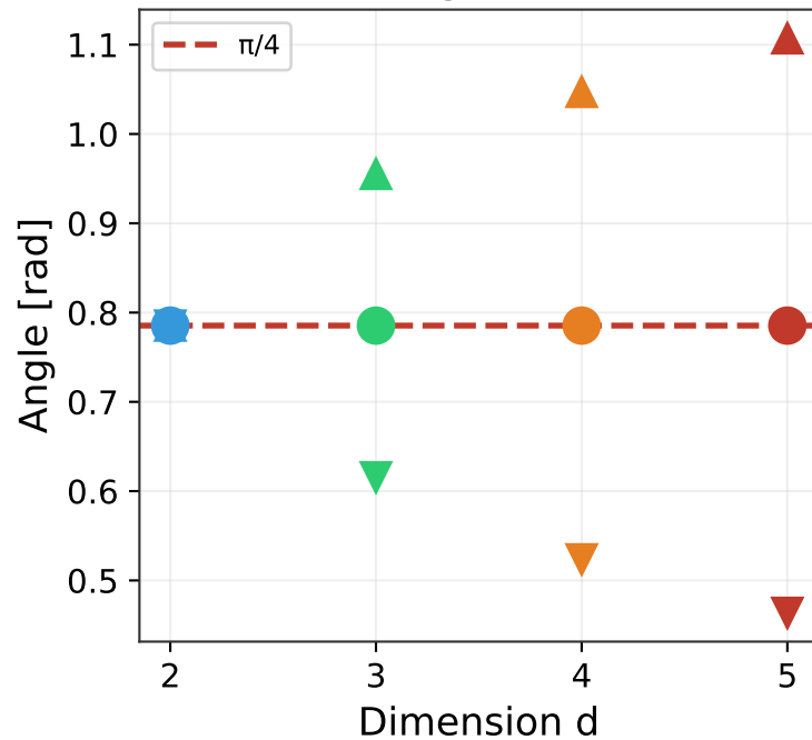
(b) Angles \rightarrow \pi/4
