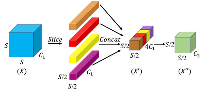
Fig. 4. SPD-Conv module structure.
