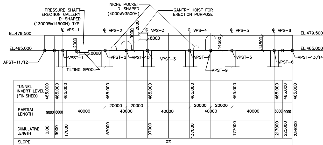
LONGITUDINAL SECTION
