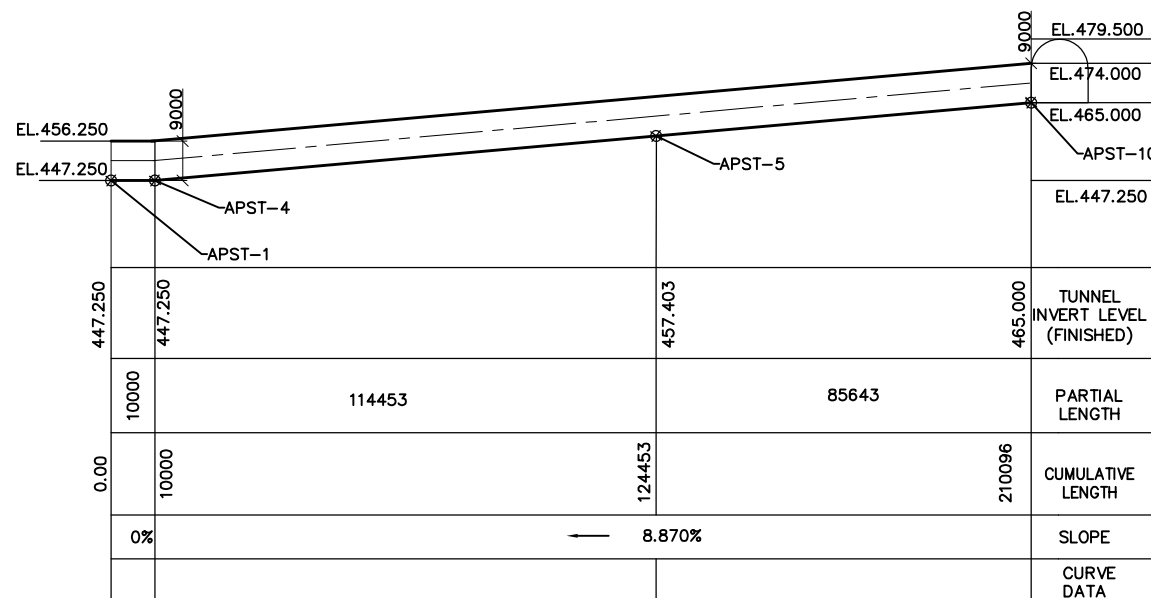
LONGITUDINAL SECTION
