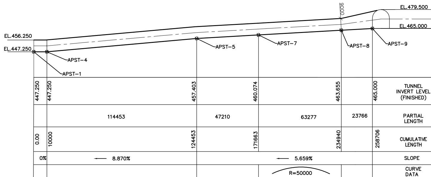
LONGITUDINAL SECTION
