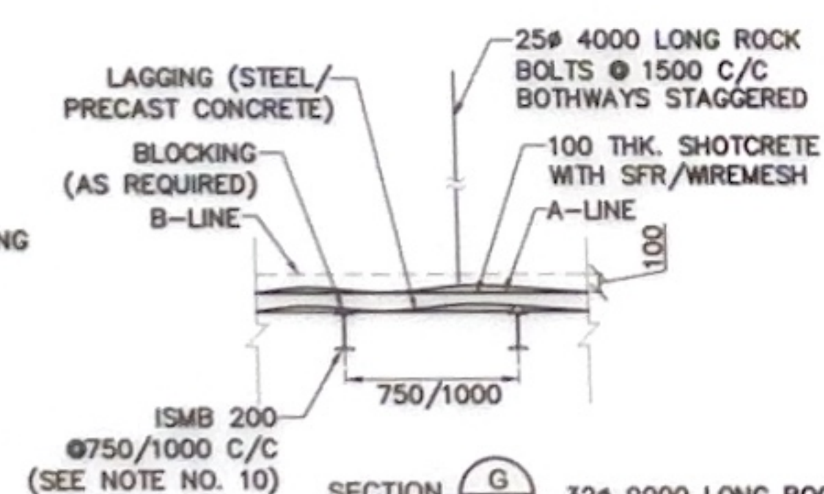
SECTION (G) (NTS)
