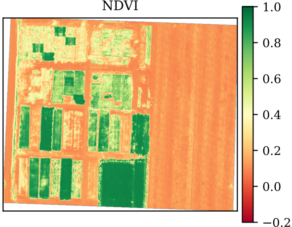
NDVI
