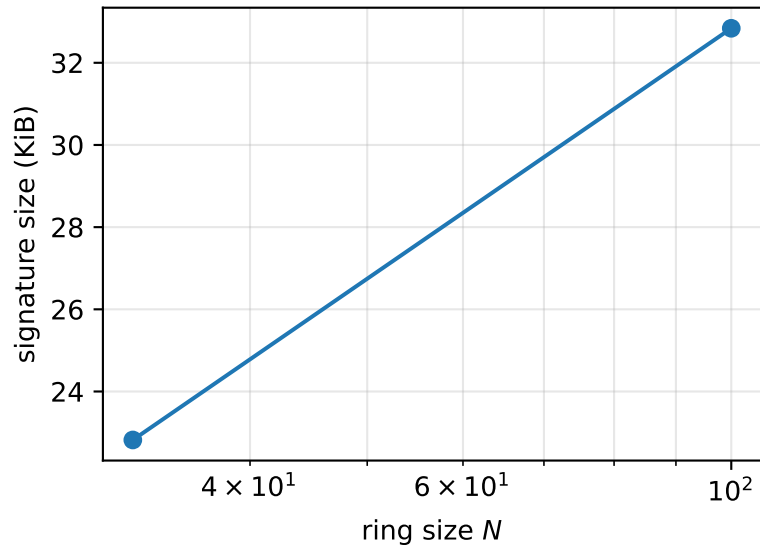
RS-alone (T=1): sig size vs N
