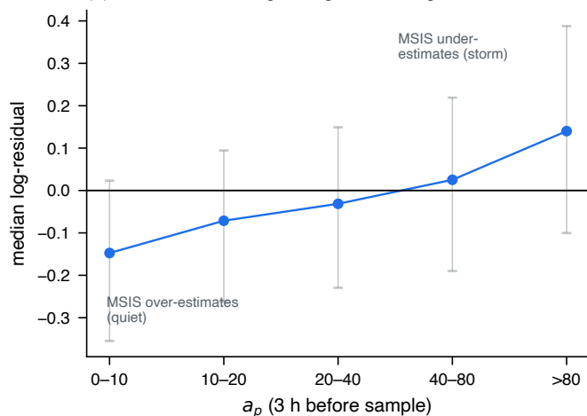
(d) Offset varies with geomagnetic forcing
