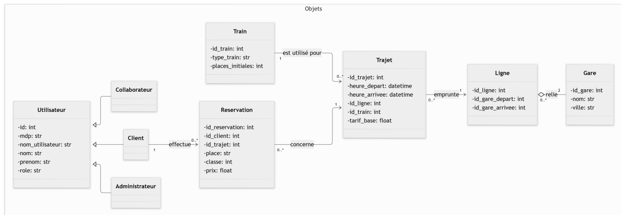
FIGURE 10 : Diagramme de classes : objets
