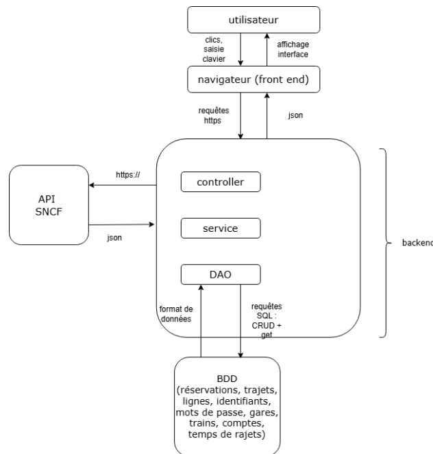
FIGURE 2 : Diagramme d'architecture de l'application
