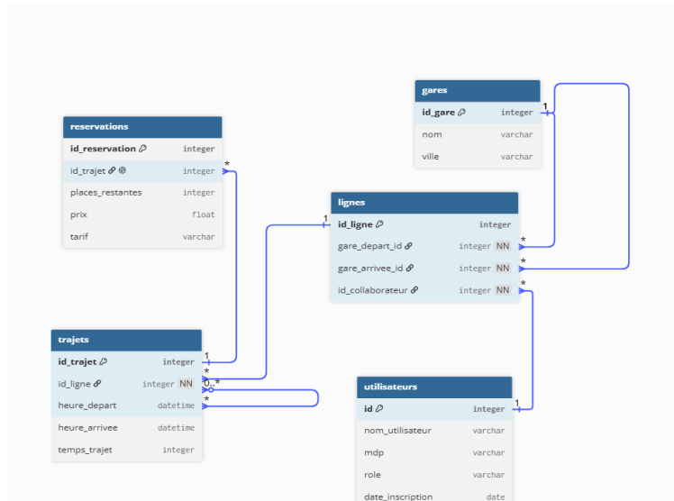
FIGURE 9 : Diagramme de base de données
