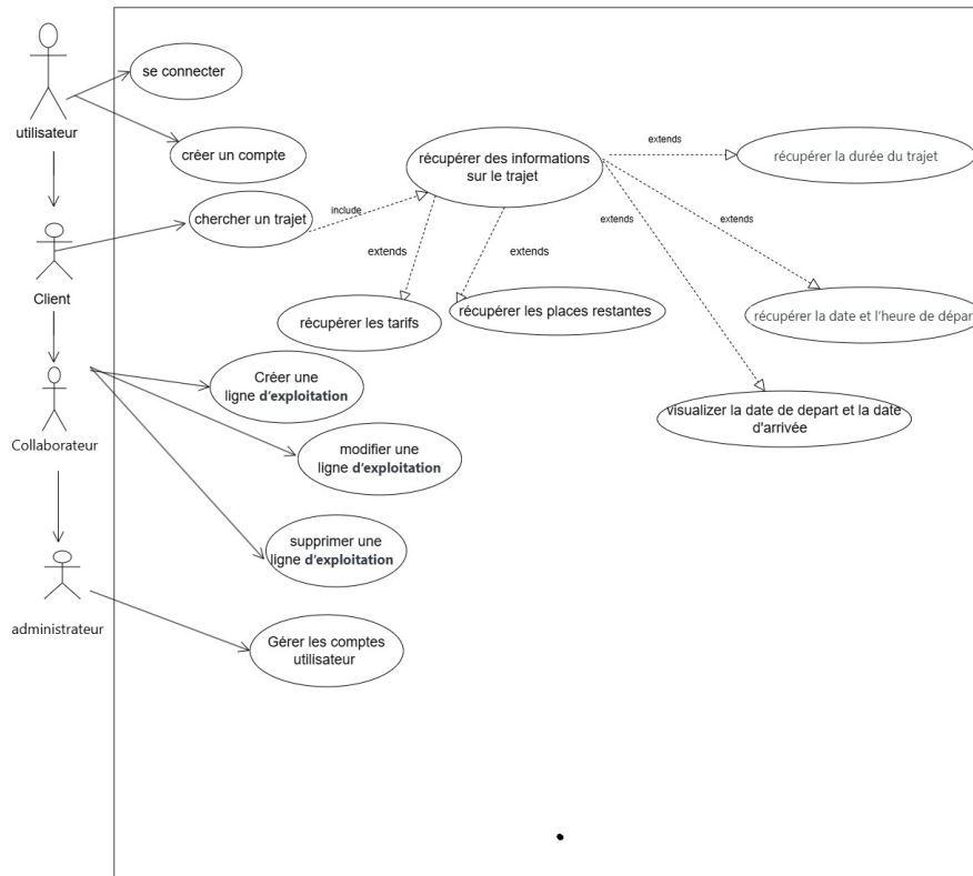
FIGURE 3 : Diagramme de cas d'utilisation
