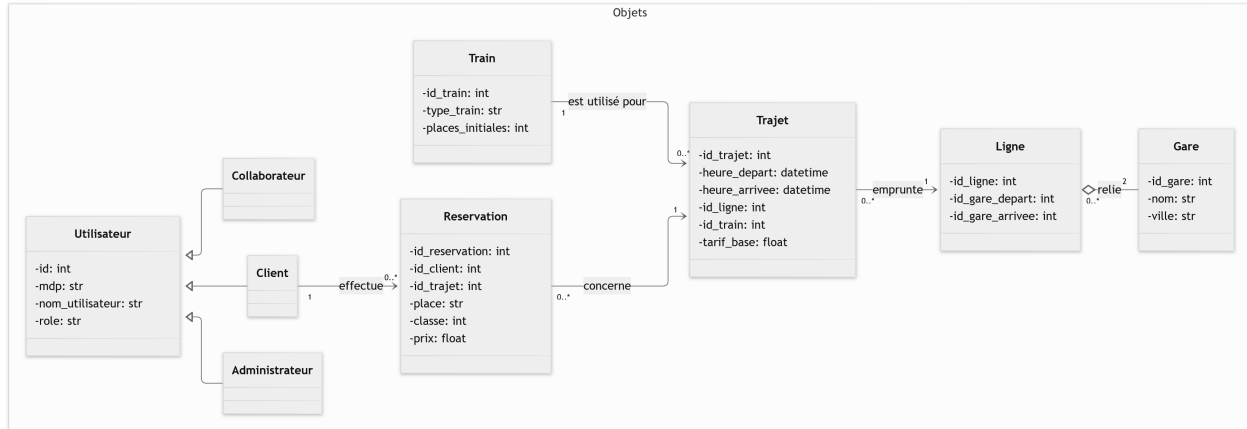
FIGURE 10 : Diagramme de classes : objets
