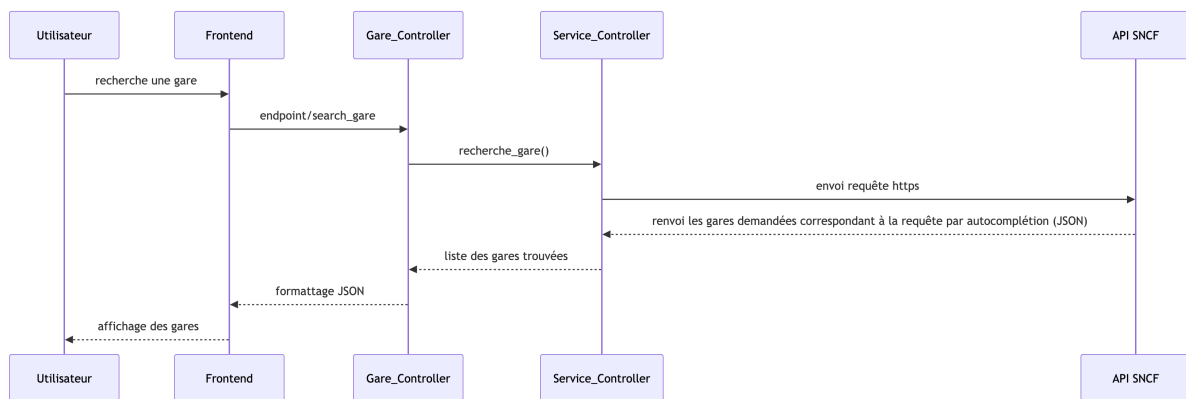
FIGURE 7 : Diagramme de séquence : rechercher une gare
