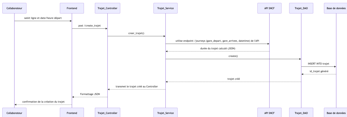
FIGURE 8 : Diagramme de séquence : création de trajet
