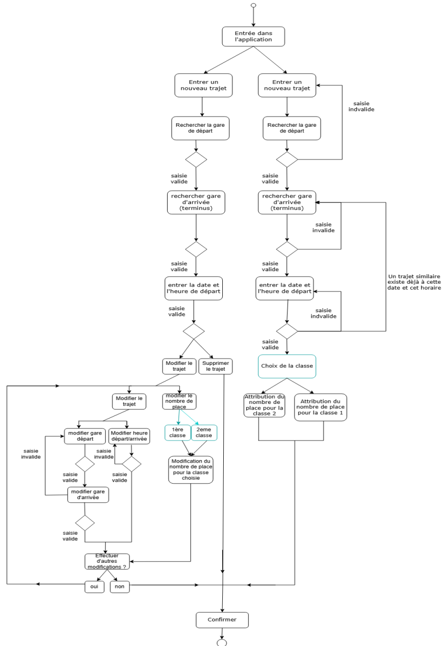
FIGURE 6 : Diagramme d'activité du collaborateur
