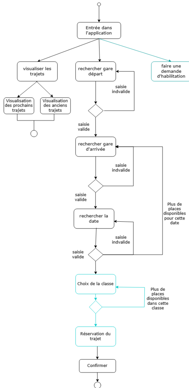
FIGURE 5 : Diagramme d'activité du client
