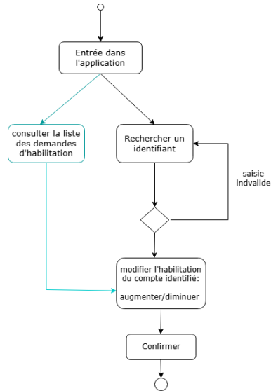
FIGURE 4 : Diagramme d'activité de l'administrateur
