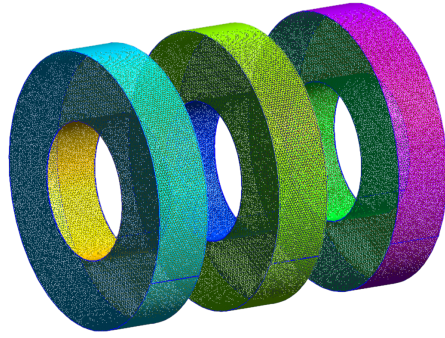
FIGURE 3.3 – Maillage de lentille de Einzel avec Gmsh
