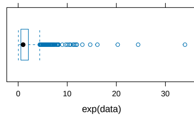
(d) Boxplot
