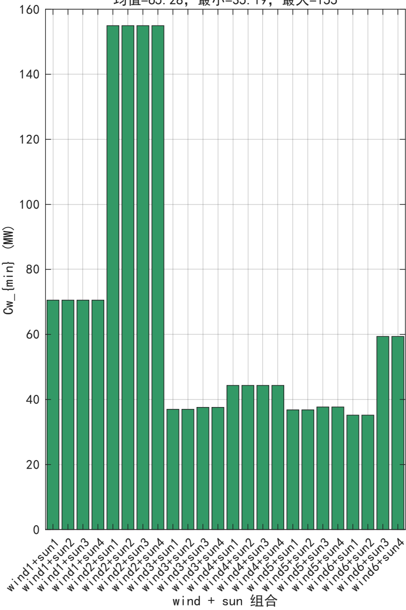
最小风电装机容量 Cw (MW) 均值=65.28, 最小=35.19, 最大=155
