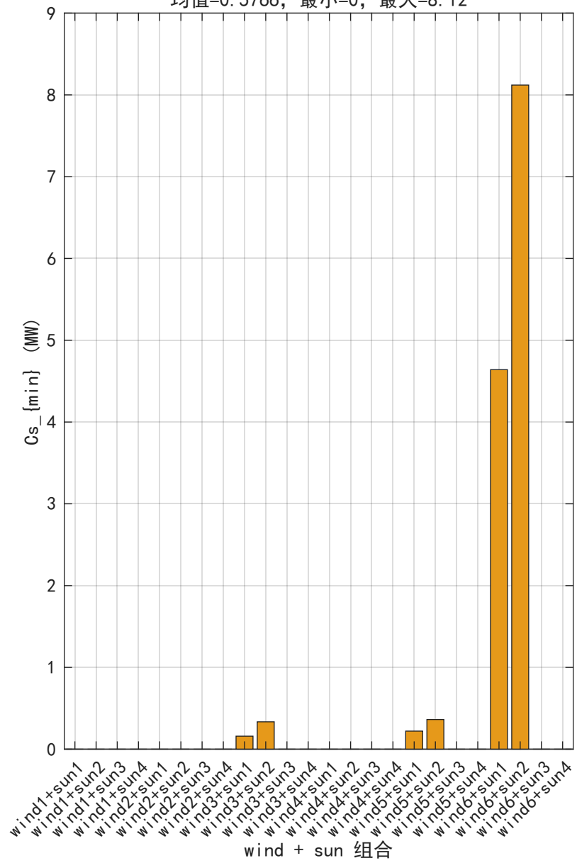
最小光电装机容量 Cs (MW) 均值=0.5766, 最小=0, 最大=8.12
