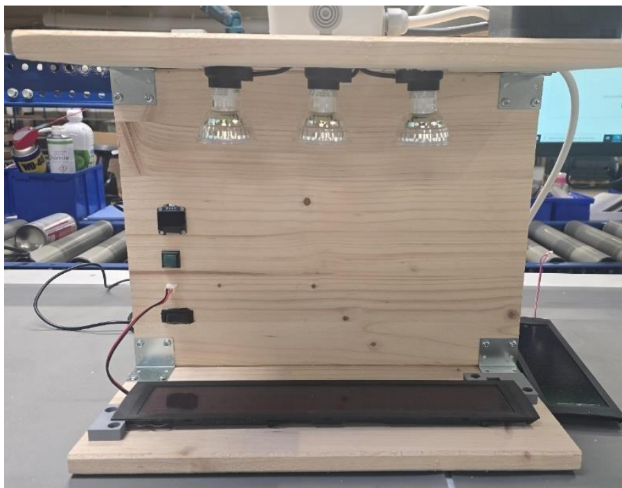
Figure 20 Banc de test automatisé et terminé
