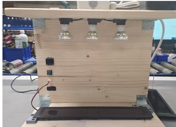
Figure 20 Banc de test automatisé et terminé
