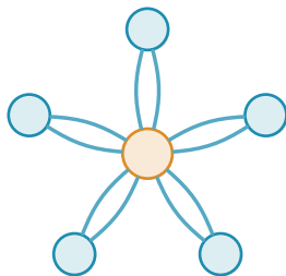
multigraph star
