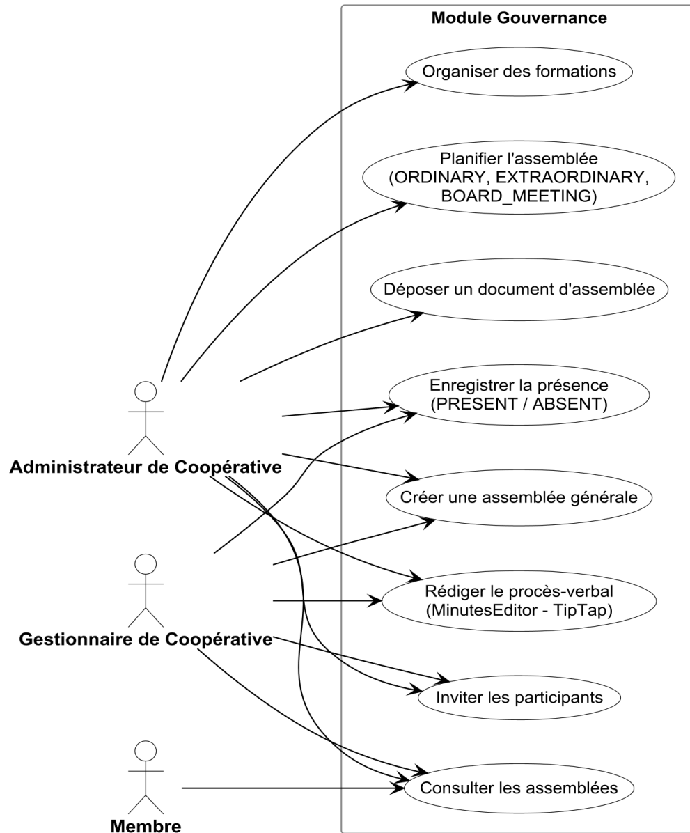
Figure 13 : Diagramme illustrant les cas d'utilisation du module Gouvernance.
