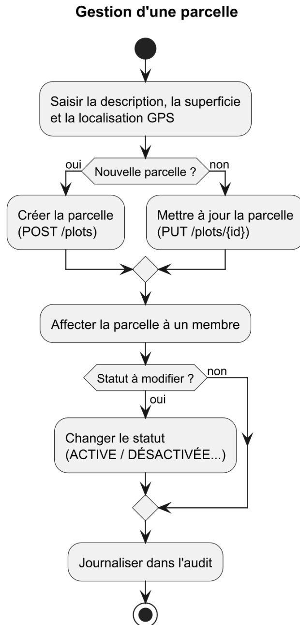
Figure 6 : Diagramme illustrant le processus de gestion des parcelles.
