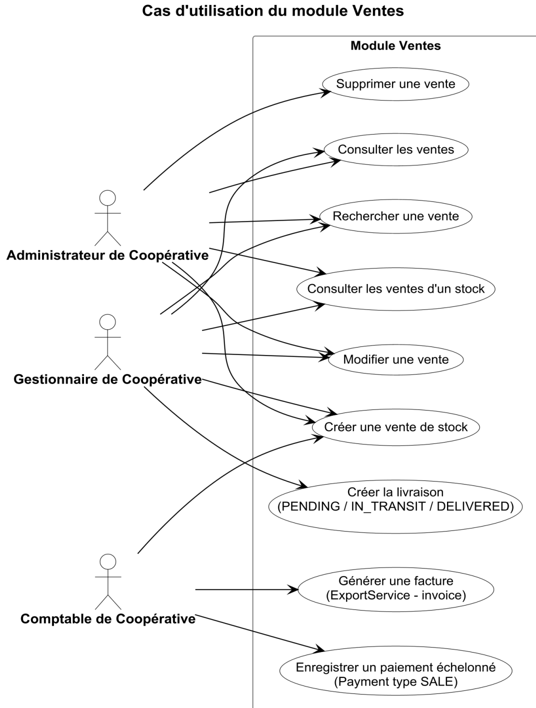
Figure 17 : Diagramme illustrant les cas d'utilisation du module Ventes.
