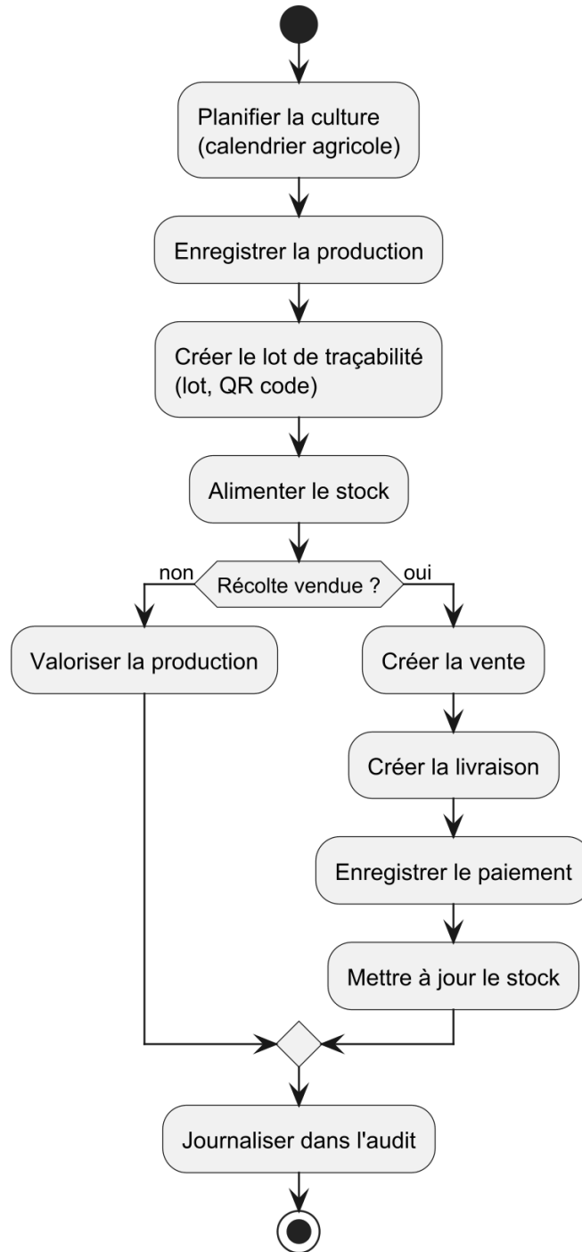
Figure 10 : Diagramme illustrant le cycle de production et de vente.
