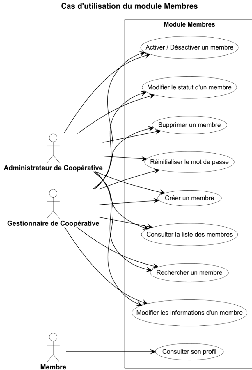
Figure 3 : Diagramme illustrant les cas d'utilisation du module Membres.
