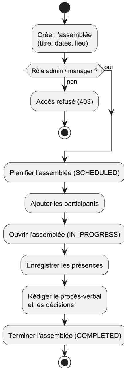
Figure 14 : Diagramme illustrant le processus d'organisation d'une assemblée générale.
