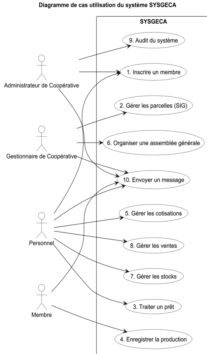
Figure 2 : Diagramme de cas d'utilisation du système SYSGECA.
