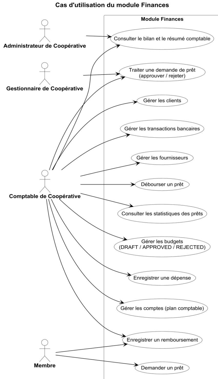
Figure 7 : Diagramme illustrant les cas d'utilisation du module Finances.
