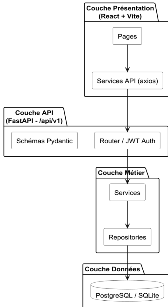
Figure 1 : Schéma illustrant l'architecture en couches du système SYSGECA.
