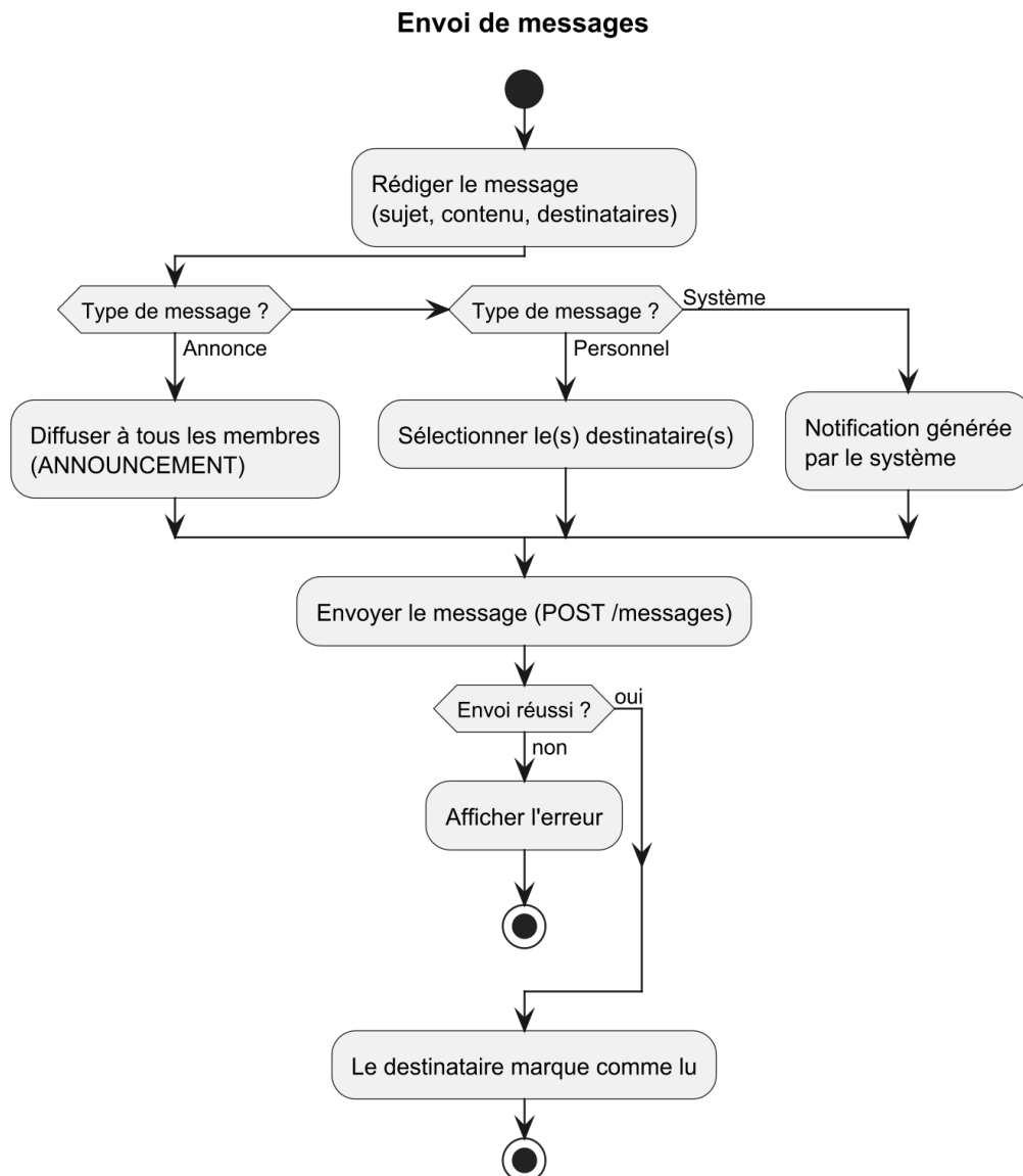
Figure 22 : Diagramme illustrant le processus d'envoi de messages.
