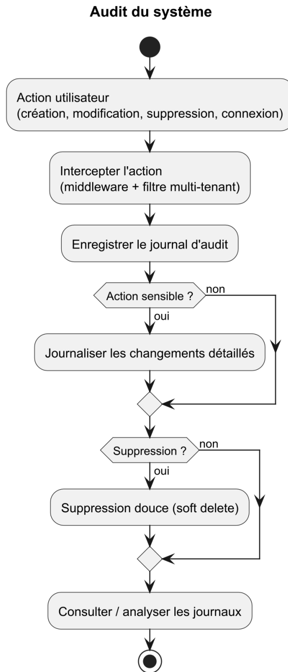
Figure 20 : Diagramme illustrant le processus d'audit du système.
