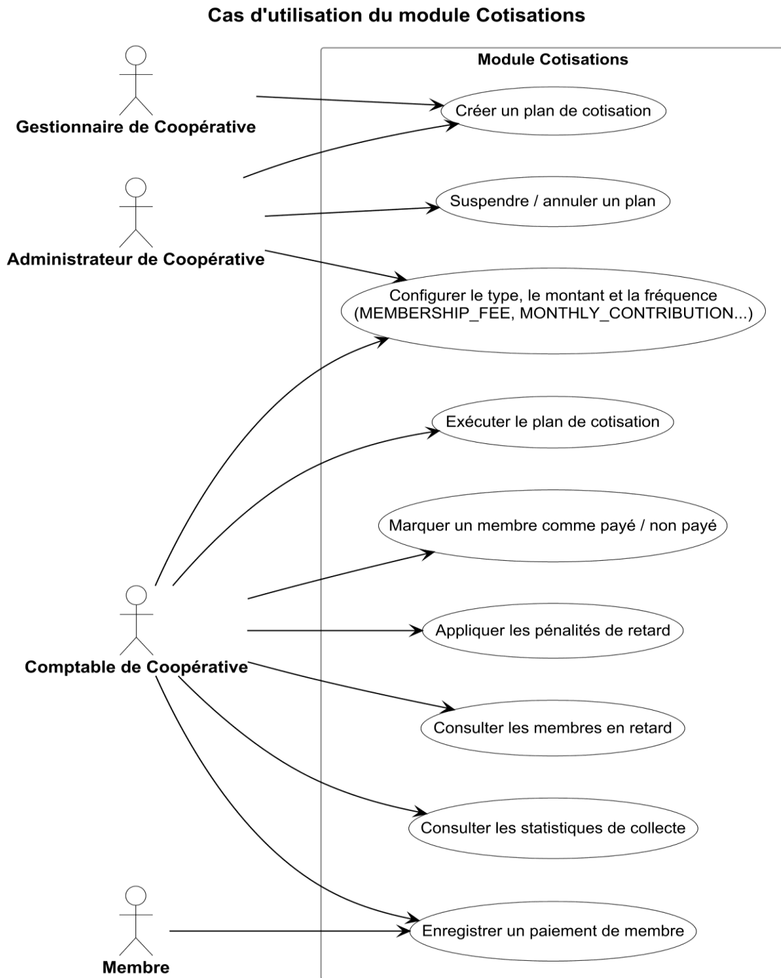
Figure 11 : Diagramme illustrant les cas d'utilisation du module Cotisations.
