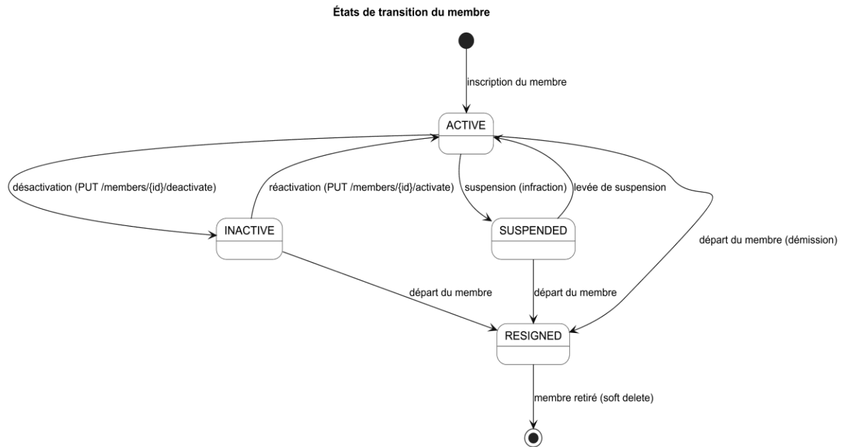
Figure 40 : Diagramme illustrant les états de transition du membre.
