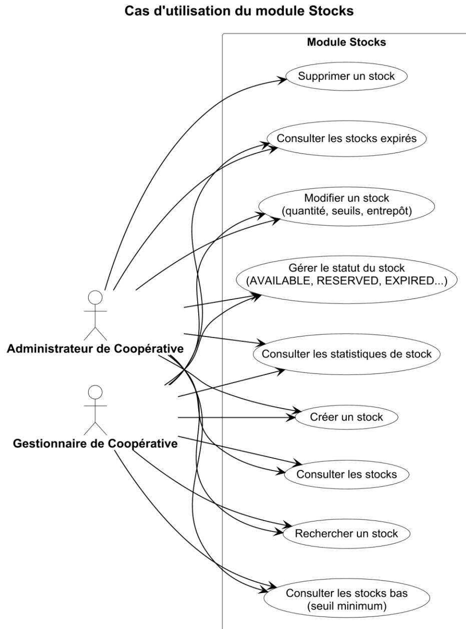
Figure 15 : Diagramme illustrant les cas d'utilisation du module Stocks.
