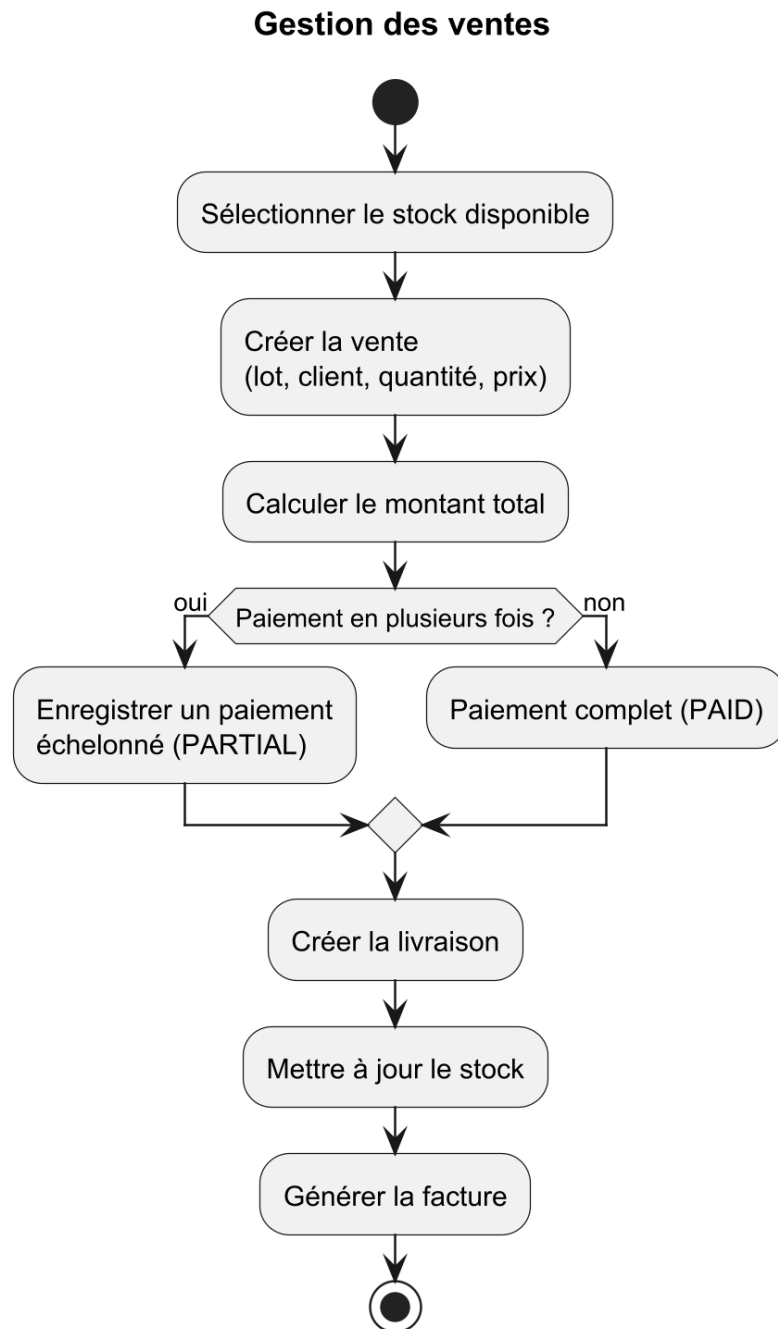
Figure 18 : Diagramme illustrant le processus de gestion des ventes.
