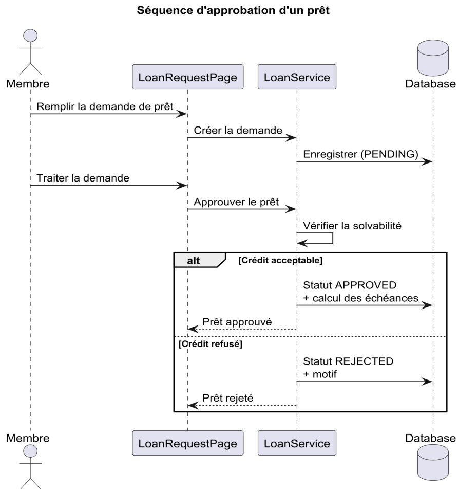
Figure 27 : Diagramme illustrant la séquence d'approbation d'un prêt.
