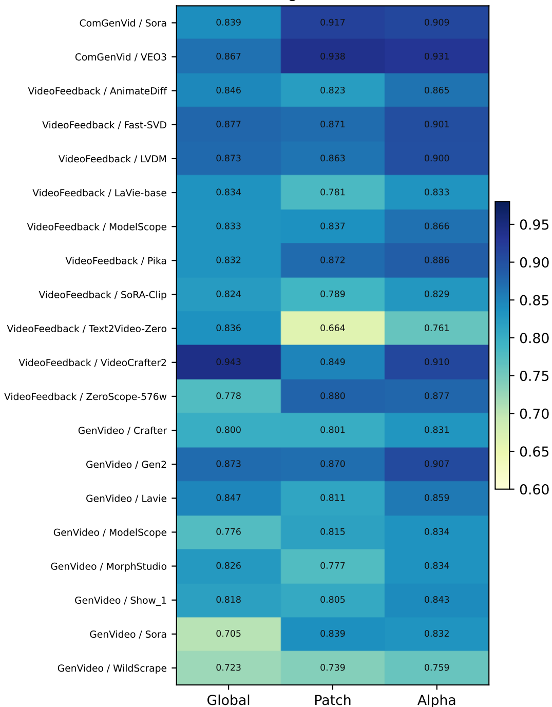
Per-generator AUC
